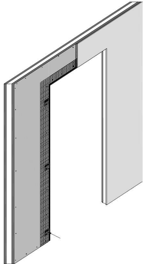
Detail/Dettaglio/Détail K
